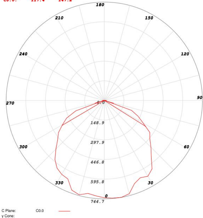
Plane [50%Ang.] [10%Ang.] 极坐标配光曲线 C0.0: 117.4 147.2
